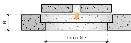
SEZIONE
